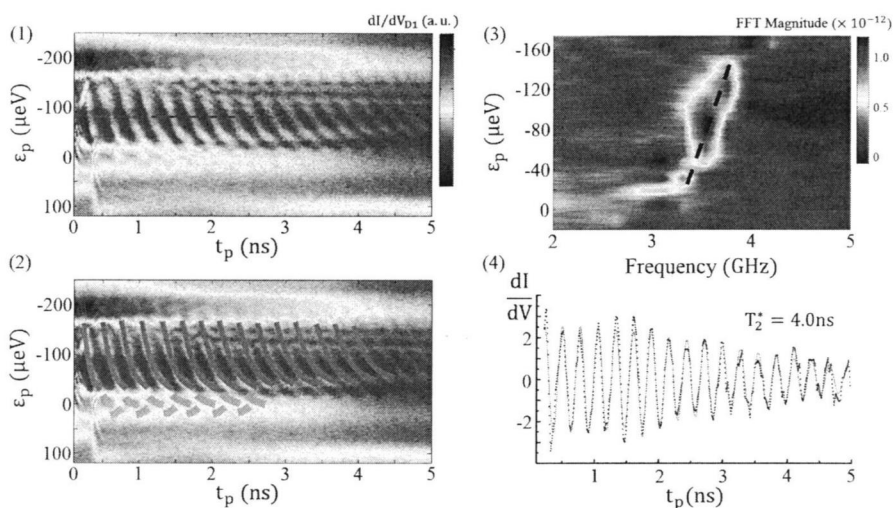
图 6.5 (1)、(2)QPC 微分电导随脉冲持续时间 t_p 和失谐量 \epsilon 的变化关系。(3) 对 (1) 中数据做傅里叶变换后得到振荡频率随 \epsilon 的变化关系。(4) 图 (1) 中虚线处提取的振荡曲线，拟合得到 T_2^* = 4.0\text{ ns} 。
