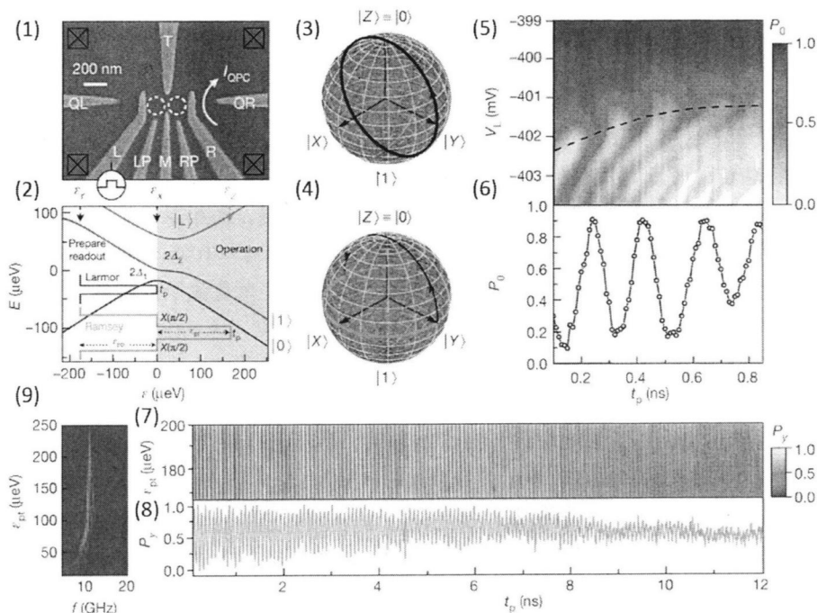
图 4.3 (1)Si/SiGe 双量子点样品结构图。(2) 根据实验数据得到的能级结构图。(3) \sigma_x 操作示意图。(4) \sigma_z 操作示意图。(5) 测量得到的 Larmor 振荡结果。(6) 黑色虚线处提取的数据曲线。(7) 实验测得的 Ramsey 干涉结果。(8) Ramsey 相图中提取的数据曲线。(9) 将 (7) 中数据做傅里叶变换得到 Ramsey 振荡随失谐量变化关系。(图片引自文献 [37])
