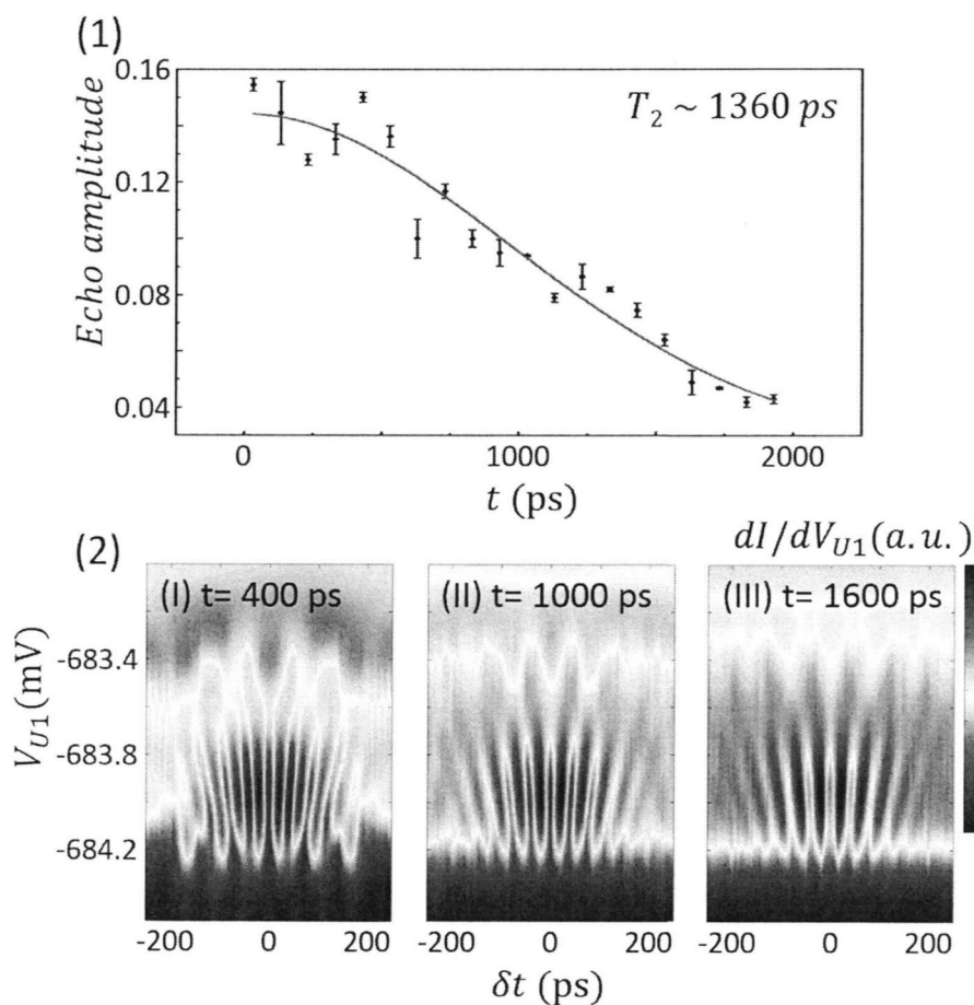
图 3.12 (1) 从实验结果提取的 echo 幅度随总演化时间 t 的变化关系，从中拟合出非均匀消相干时间 T_2 = 1360 \pm 400 ps。 (2) 利用实验数据模拟得到的 echo 过程。
