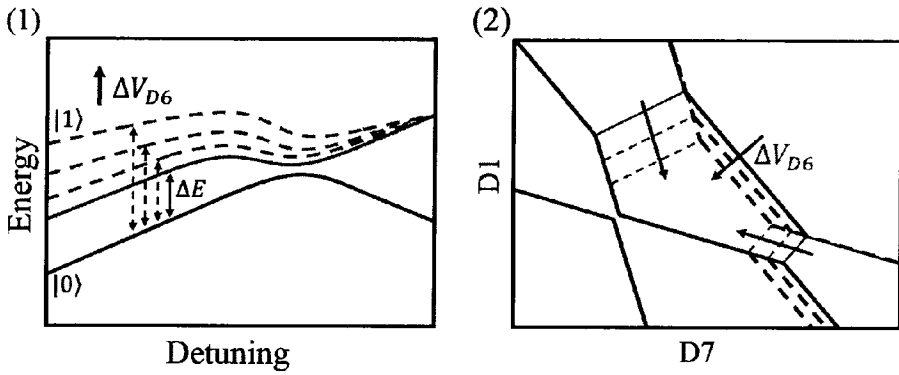
图 6.8 (1) 三点中构造的平行能级结构示意图。(2) 调节 V_{D6} 时, 三量子点电化学势变化示意图。
